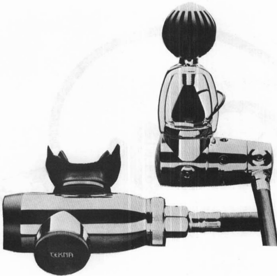
Tekna T-2100
