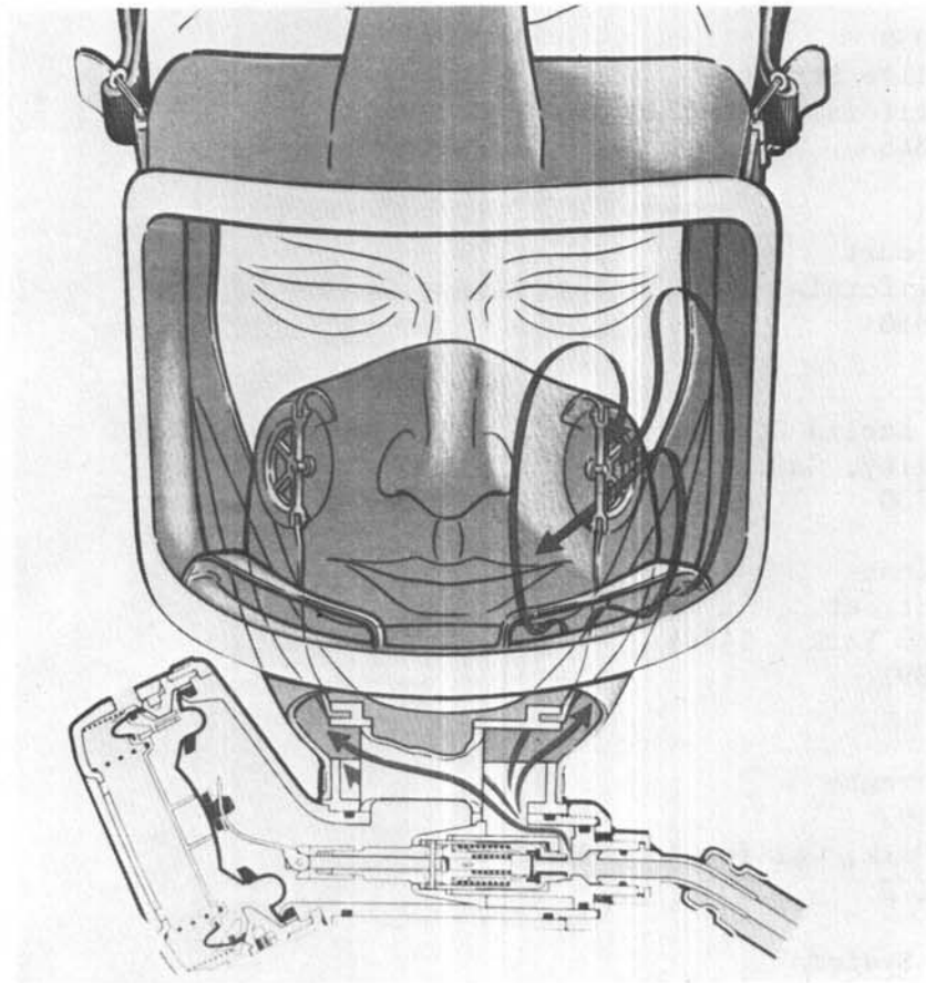
AGA Divator 324
