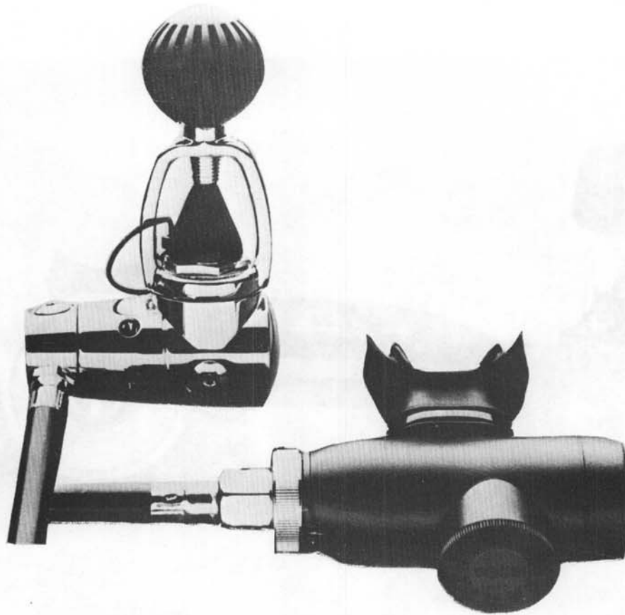
Tekna T-2100B
