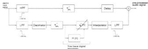
Fig. 11. Multirate non linear processor.
